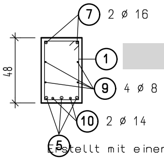
SCHNITT A-A
