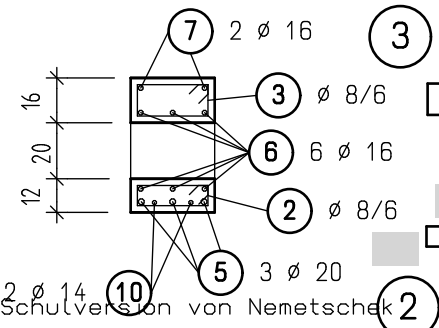
SCHNITT B-B
