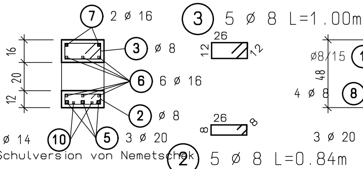
SCHNITT B-B
