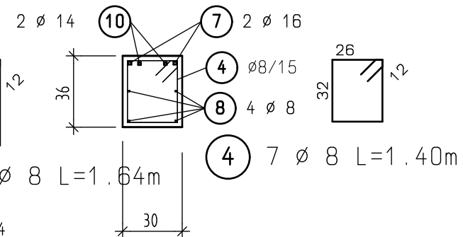
SCHNITT D-D
