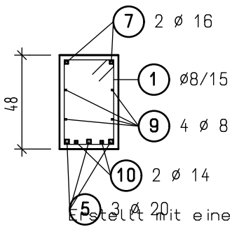
SCHNITT A-A
