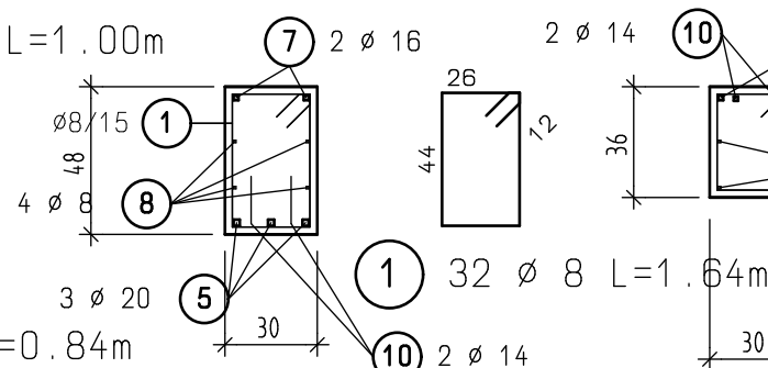
SCHNITT C-C
