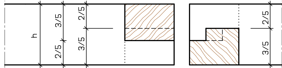
AUFRISS
