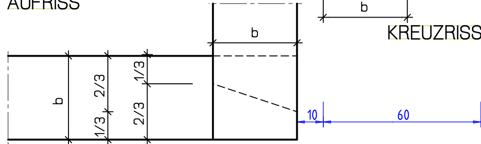
GRUNDRISSE
