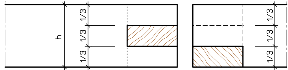
AUFRISS
