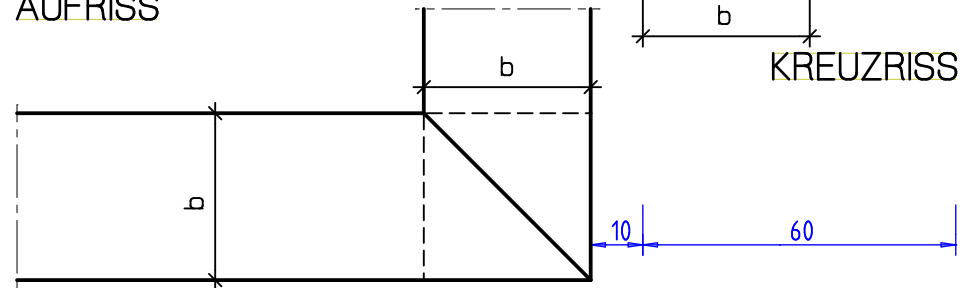
GRUNDRIS
