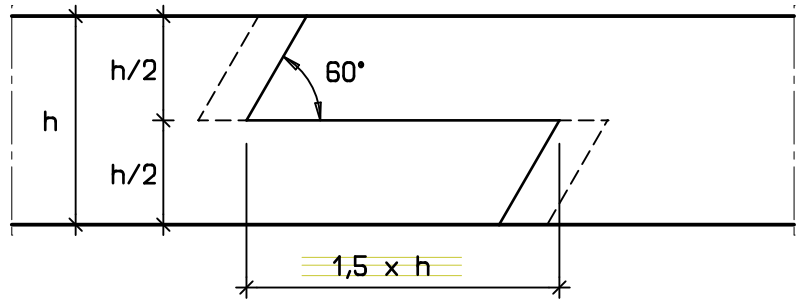
AUFRISS
