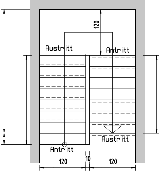
Beispiel 2 Zweiläufige Halbpodesttreppe Geschoßhöhe: 2,91m; Stufenbreite 29cm; Hauptstiege; Decke + Aufbau: 28cm
