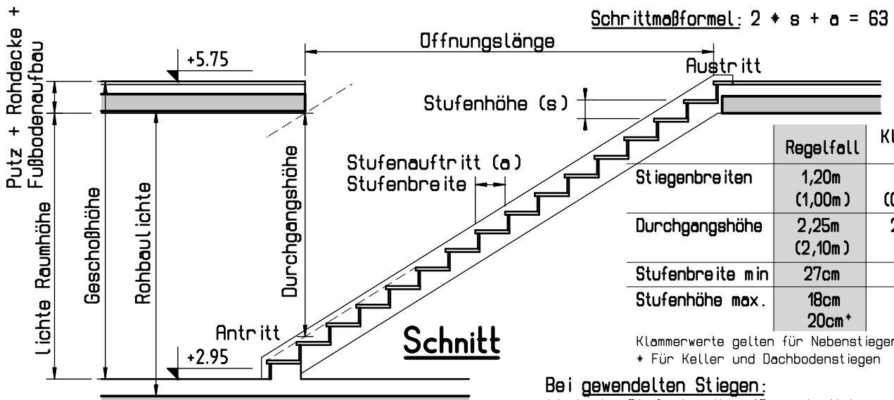
Beispiel 1 Einläufige, gerade Stiege Nebenstiege, lichte Raumhöhe: 2,50m
