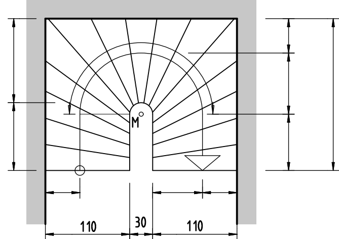
Beispiel 3 Halbgewendelte Stiege Geschoßhöhe: 2,84m; 16 Steigungen; Kleinwohnhaus; Decke + Aufbau: 32cm
